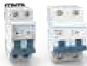
DC NO-POLARITY BREAKER 1000V 63A & 200V 125A 20-31
