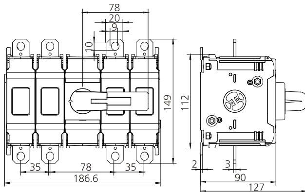
Frame EHA315:EHA-DB-22
