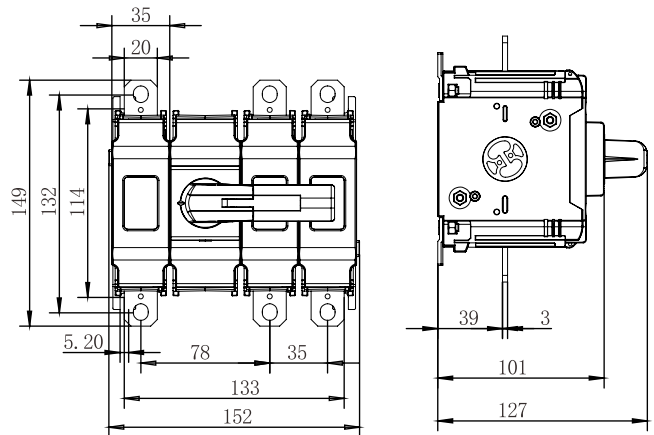
Frame EHA315:EHA-EL-02
