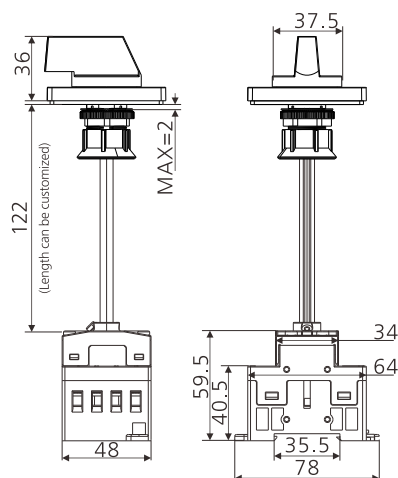
4Poles 20-40A
