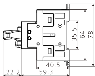
4Poles 20-40A
