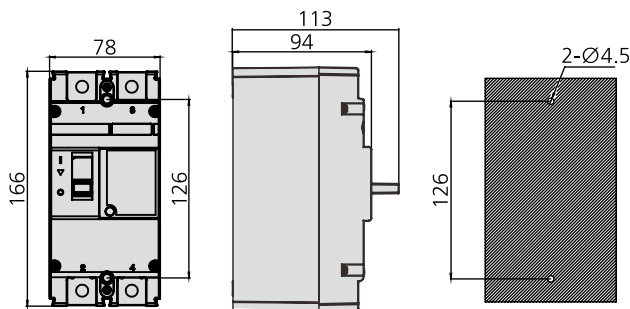
EDM3 -250
