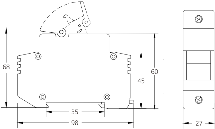
EDFHT-32/1
