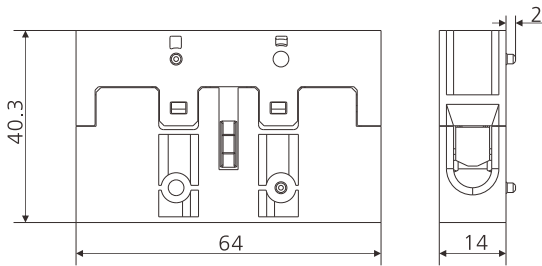
JHAC69-ACC03
