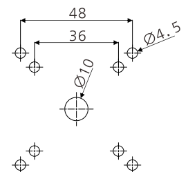
door lock hole
