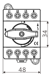
4Poles 20-40A
