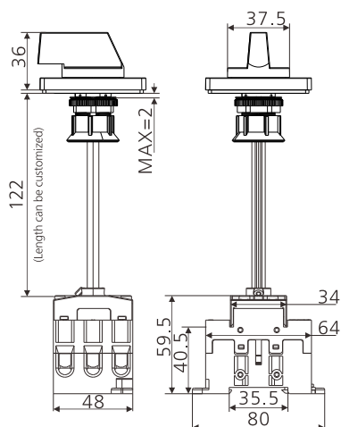
3Poles 63-80A
