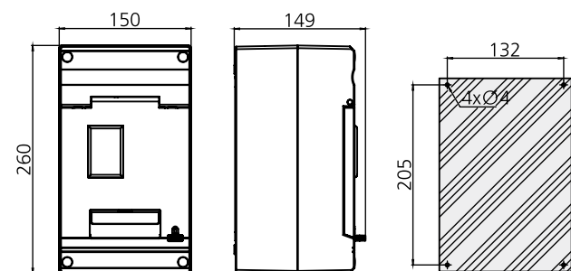
EDM3 -250/EL
