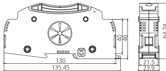
EDFHT-50/1L
