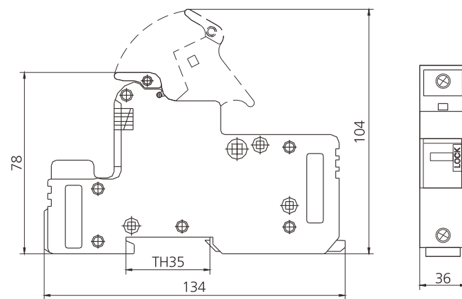
EDFHT-50W/1
